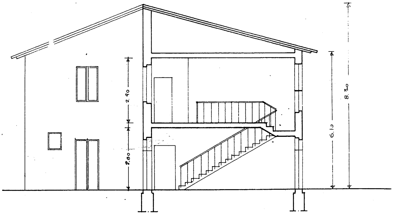
Sezione: A-B
