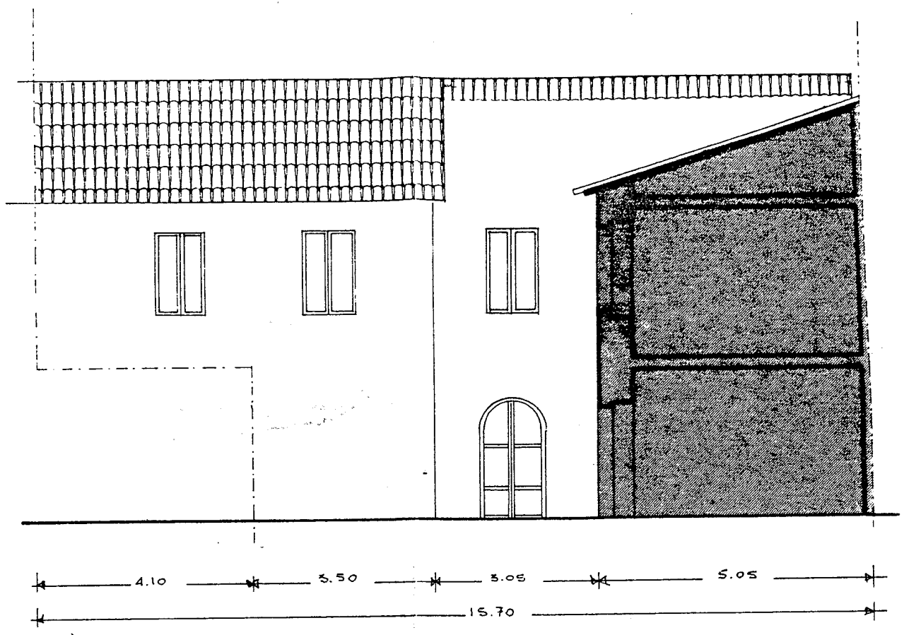
Prospetto 1
