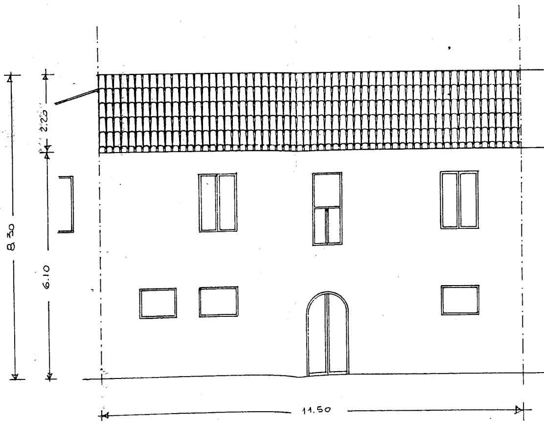
Prospetto 1
