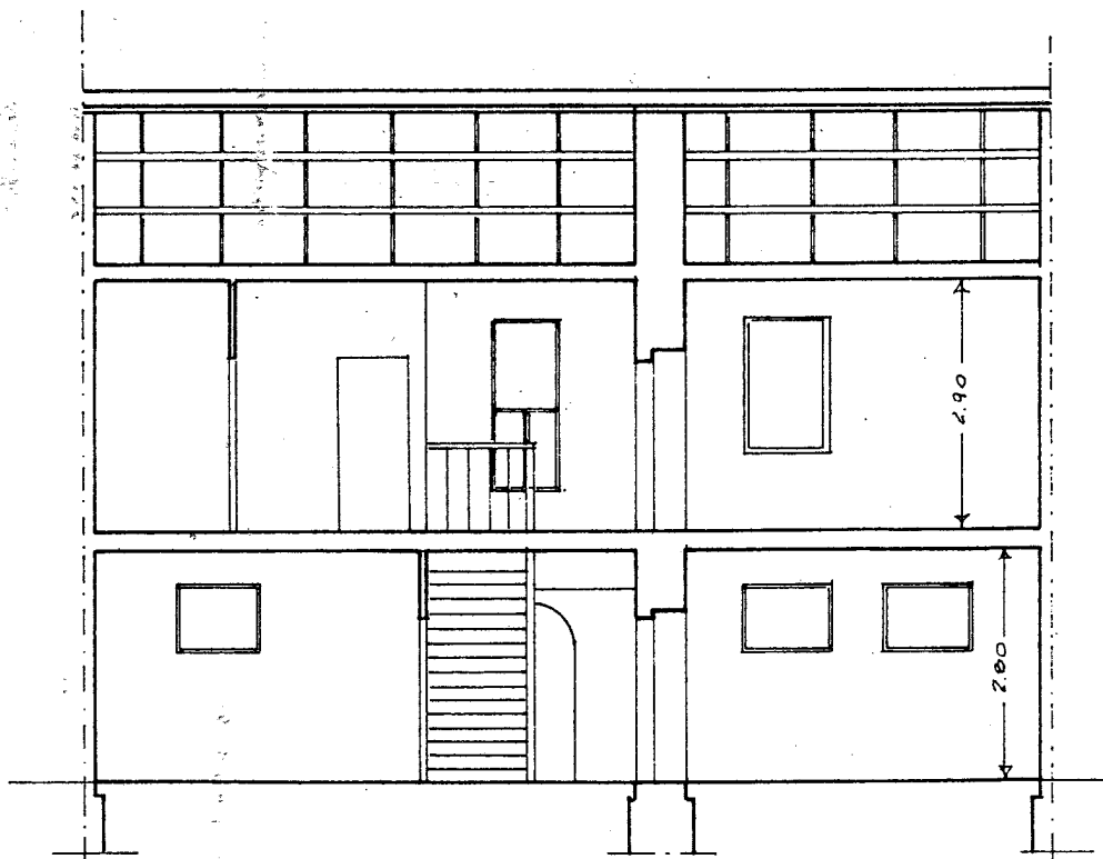
Sezione: C-D
