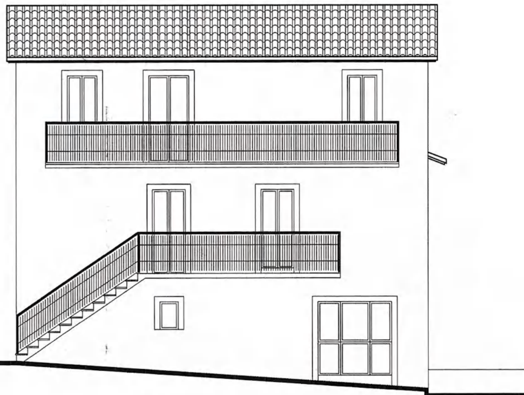
PROSPETTO SUD
