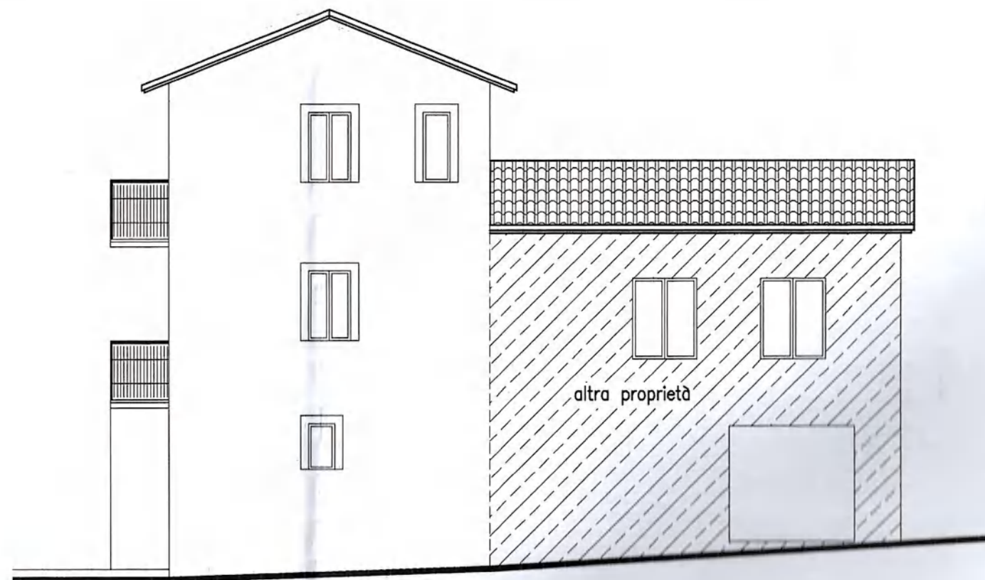
PROSPETTO EST
